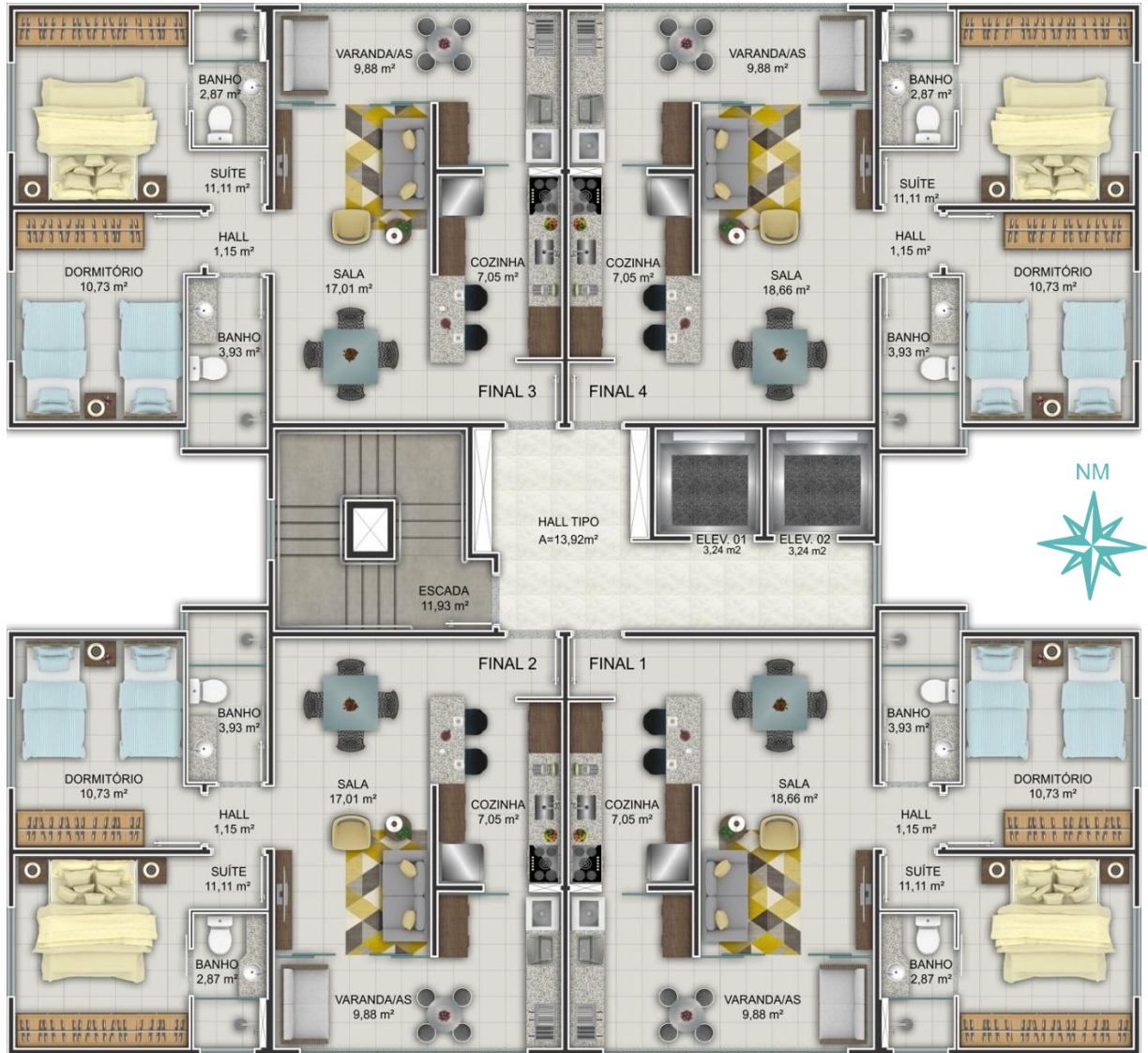
Planta Baixa Pavimento Tipo
