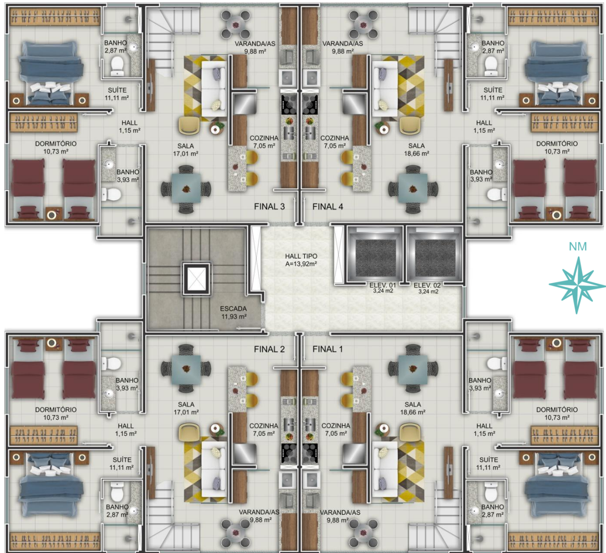
Planta Baixa Pavimento Duplex Inferior
